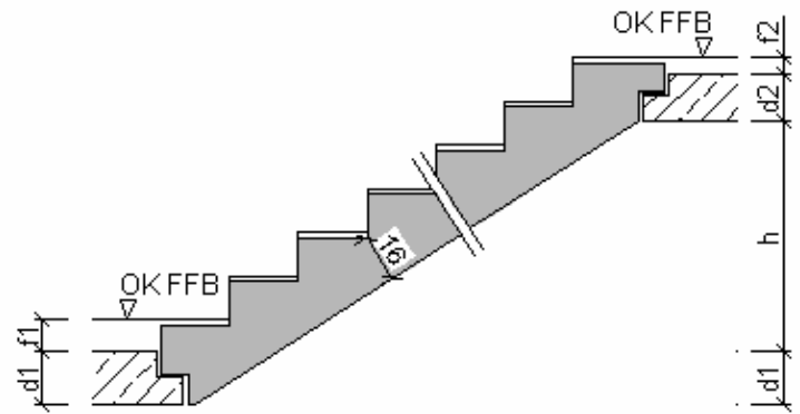
Doppelt gewendelte Treppe Typ 1 + 2 [m]
