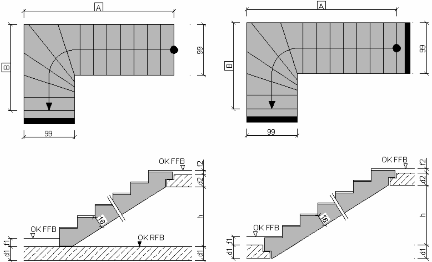
Einfach gewendelte Treppe Typ 1 [m]
